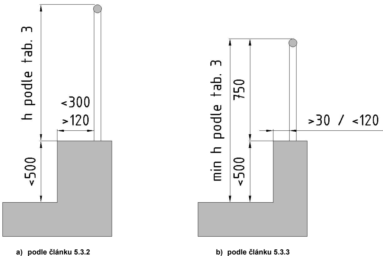
Obrázek 2 – Výška zábradlí s parapetem
