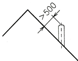
Obrázek 6 – Výška přetlakového komína od roviny střechy
