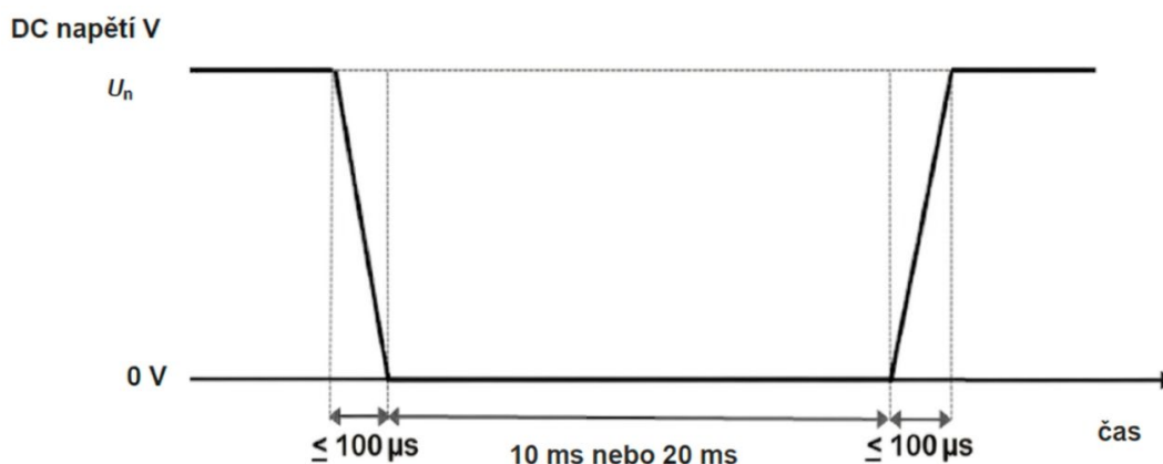
Obrázek 10 – Přerušení napájení
