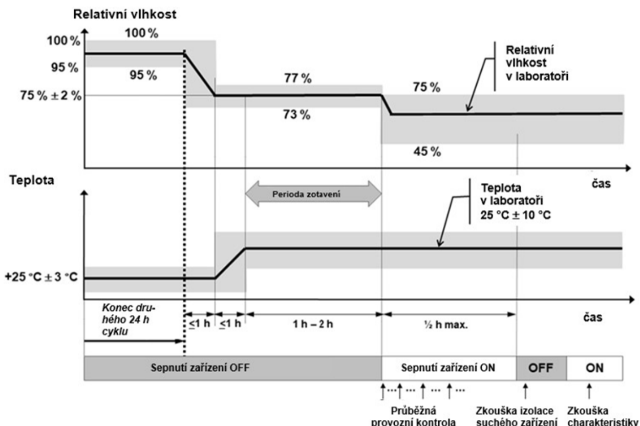
Obrázek 18 – Cyklická zkouška vlhkým teplem: Konec druhého cyklu a perioda zotavení
