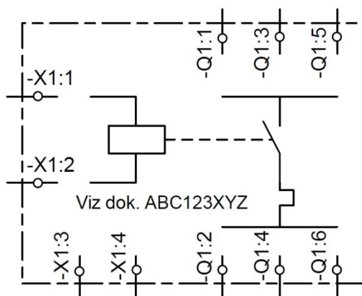
Obrázek 97 – Příklad vzorového schématu spouštěče motoru
