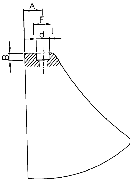
Obrázek 1 –Nástěnná pisoárová mísa s horním přítokem
