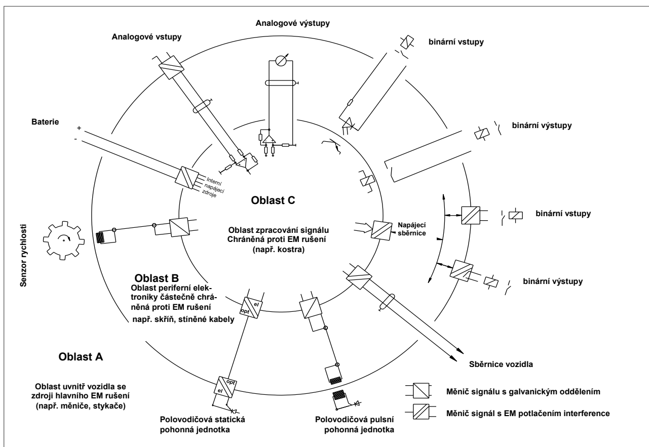
Obrázek 5 – Rozhraní systému s typickými oblastmi EMC – oblast A, B a C
